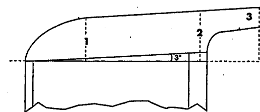
EN PLAN. - Noter l'angle de 3° auquel est calé l'ensemble du bloc balsa sculpté. Le plus simple est de décaler la nervure marginale.
