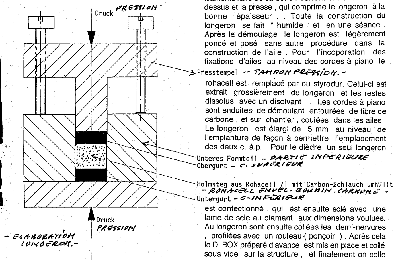
Abb. 2: Holmaufbau und Holmform
