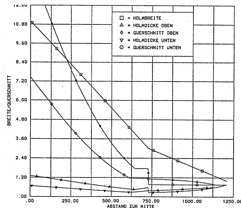
Abb. 1: Holmabmessungen
