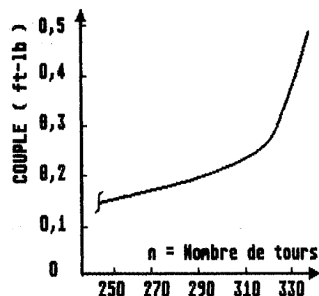
FIG 2 - Caractéristiques du moteur caoutchouc.
