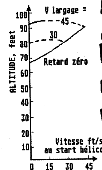
FIG 7 - Altitude suivant vitesse au start hélice
