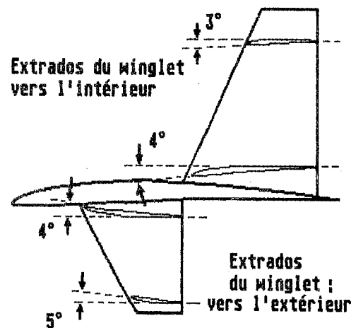
SUGGESTION pour un moto F1C
