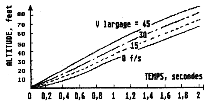
FIG 4 - Altitude obtenue, pour 4 vitesses de largage
