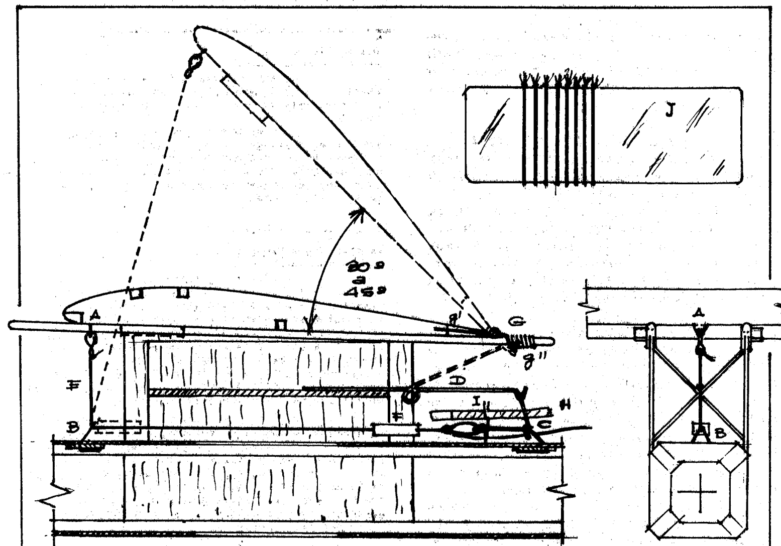
SECCION LONGITUDINAL (ESC. 1/1) VISTA FRONTAL
