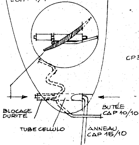
DÉTAIL PIED DE PALE ECH: 1/1
