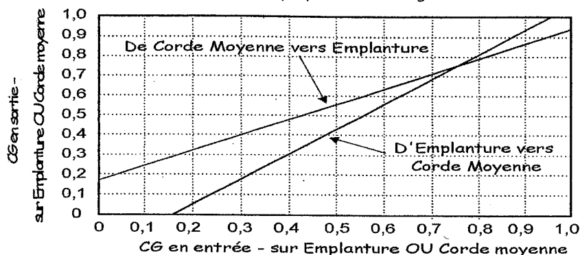
Conversion du CG entre Cordes Moyenne et Emplanture pour Aile elliptique à BF rectiligne
