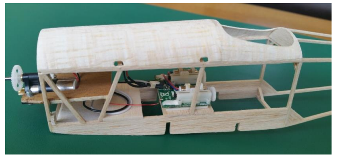
Mitsubischi 1MF3 de Philippe Lacourt inspiré du plan de Roger Aime. Envergure 36 cm, poids approximatif 40 g. L'ensemble propulsif semble venir d'un Minium 8 mm. Détails de finition en cours.....
