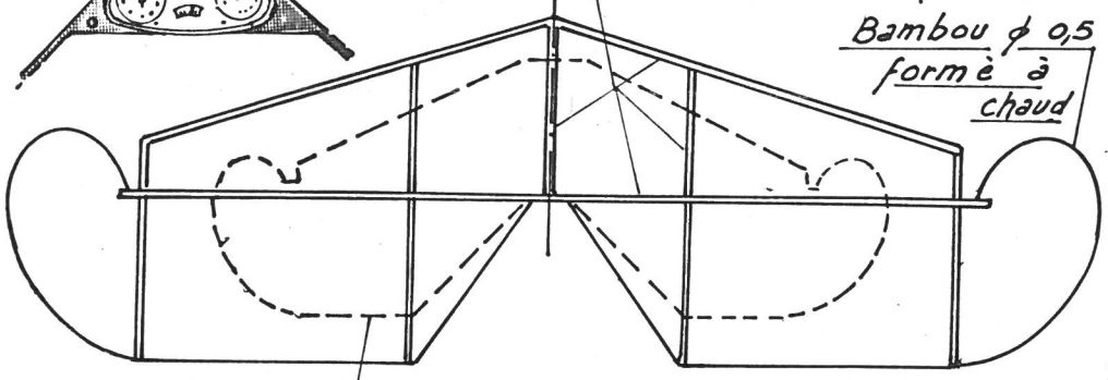
Contours à l'échelle
