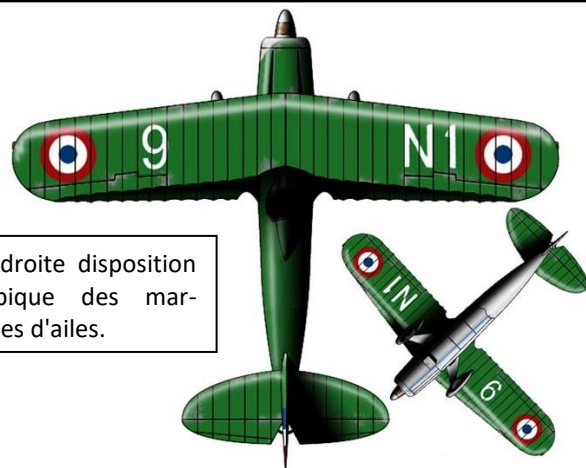
SPAD 510 n° 26 "I" du Lt Ozanne, commandant de la 1 re escadrille du GC I/7, Dijon juin 1938.
