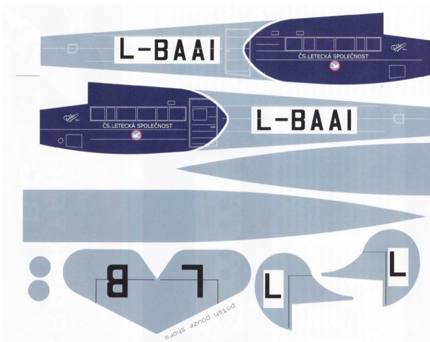
Fokker L-VIIa - potah trupu a ocasech ploch (vřídlo je stříkané)
