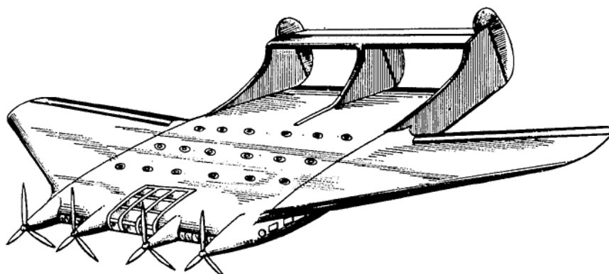
BURNELLI GB 177 Projet tardif de transport militaire.
