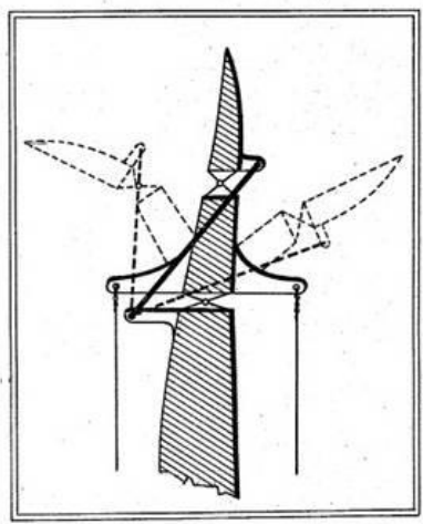
L'aileron de l'avionnette Peyret-Nessler.
