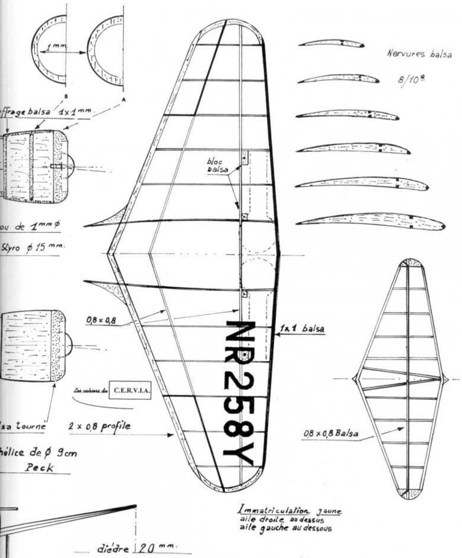
Howard Hughes Racer H1 "Pistachio" Dessiné par Roger Aime. Doc. Benno Sabel D. Bill Warner U.S.A. le 11/04/2005
