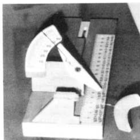
Rapporteur contrôleur de pas d'hélice, une réalisation de F. MANIERI ( p. 611 )
