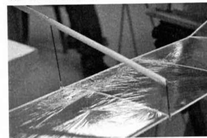
FID – mâts en fibre de carbone
