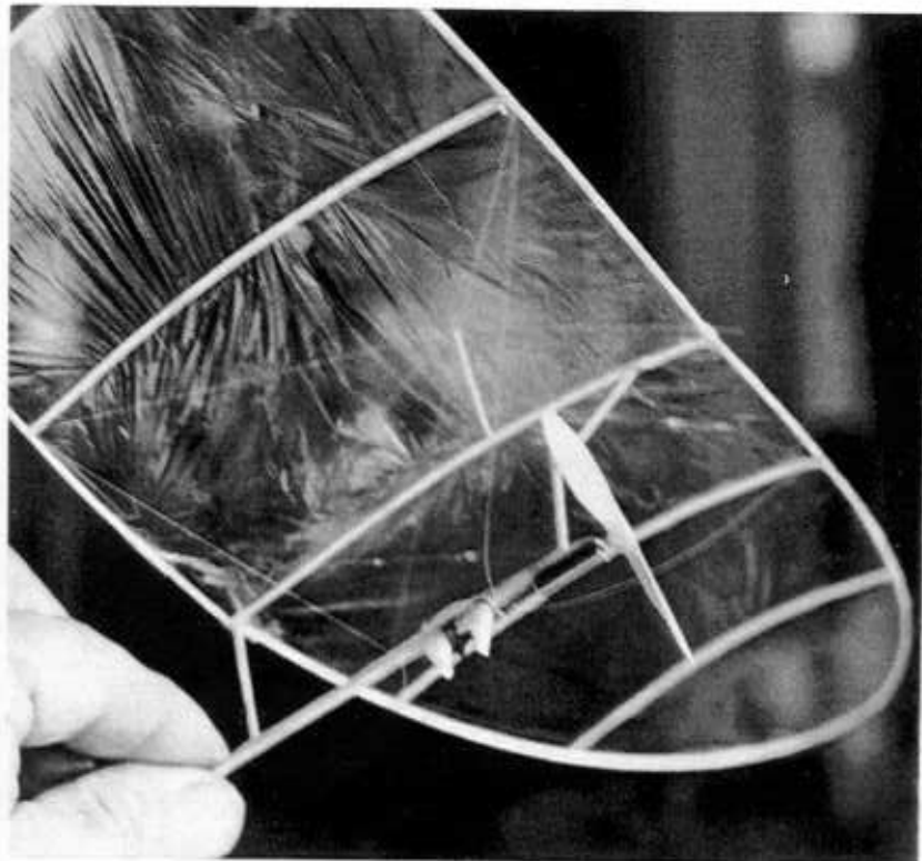
UN M.A.V.? Non, c'est l'ELECTRO LIGHT d'Emmanuel FILLON : 1,6g !
